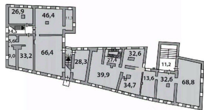
2 этаж: Площадь - 516,8 кв.м.
